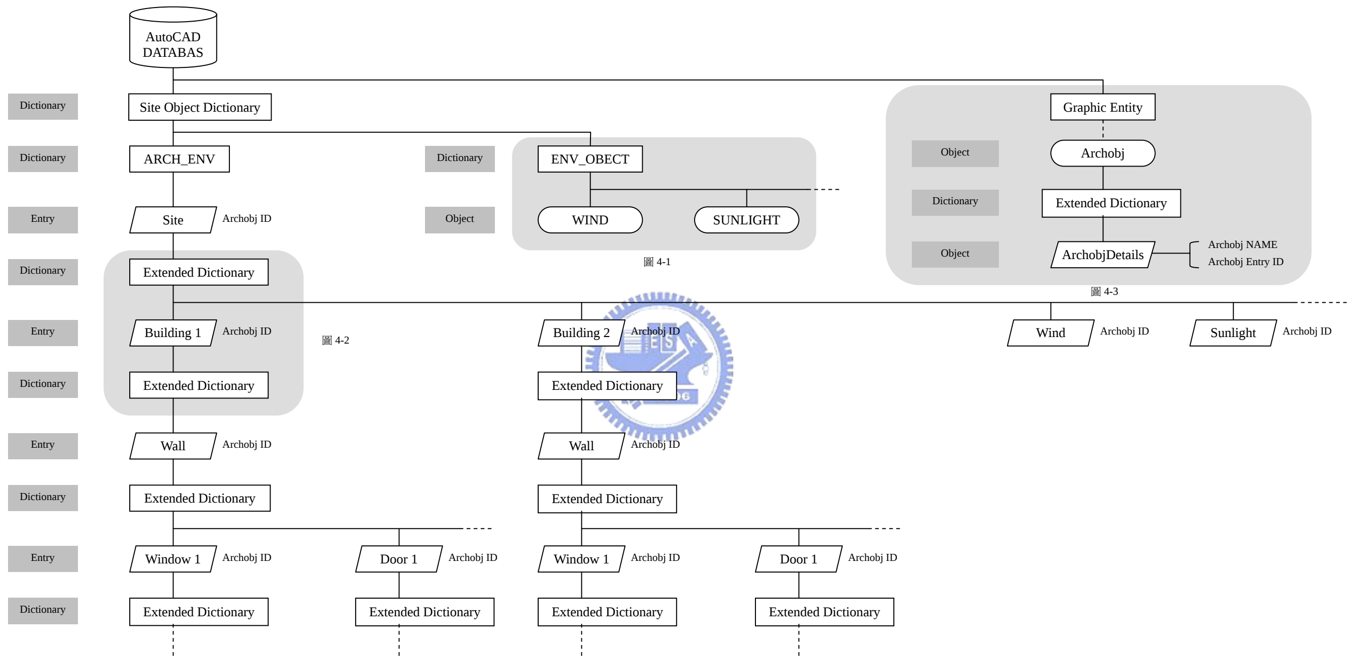
圖 4-5 輔助設計系統之階層式架構圖
