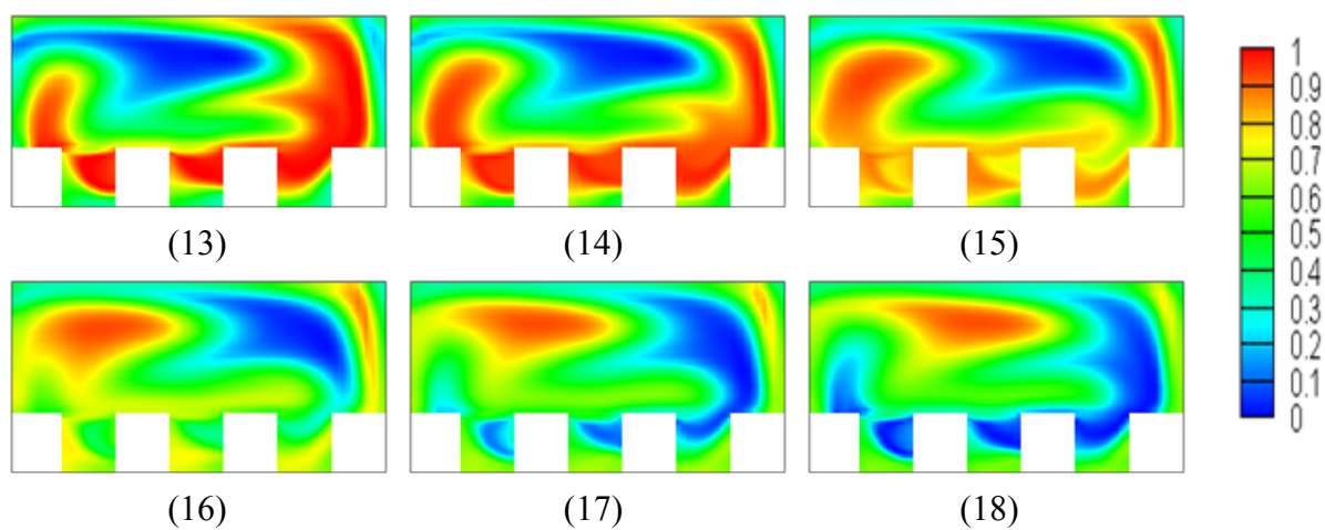
圖 4-36 SRM \alpha = 30^\circ 從入口到 1cm 之間截面濃度分佈
