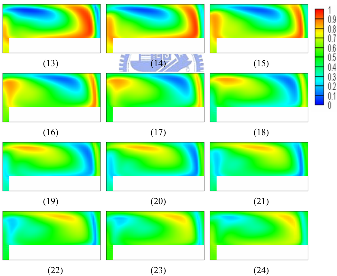
圖 4-42 SRM \alpha = 75^\circ ，下游 1~2cm 之間截面濃度分佈
