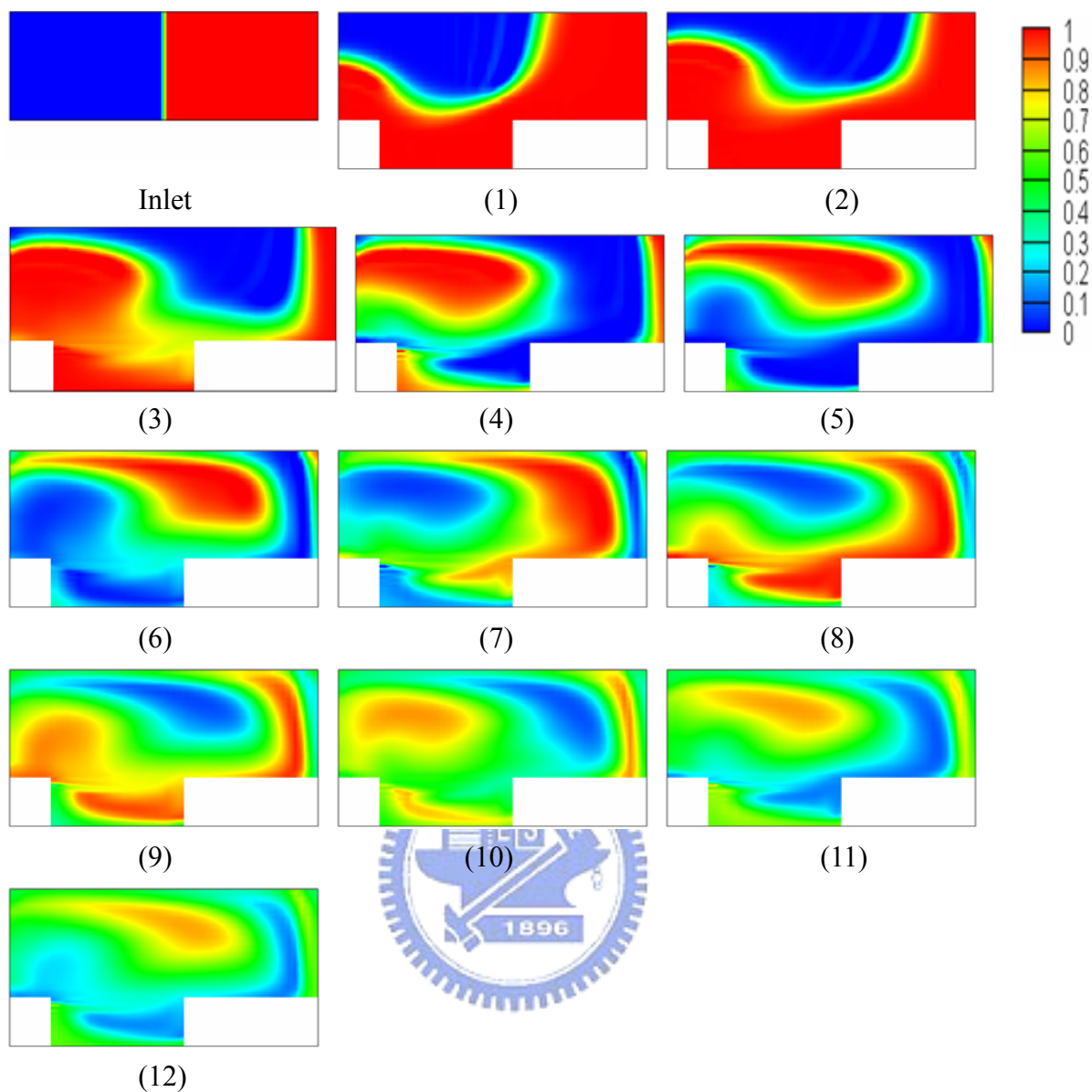
圖 4-39 SRM \alpha = 60^\circ ，入口到 1cm 之間截面濃度分佈
