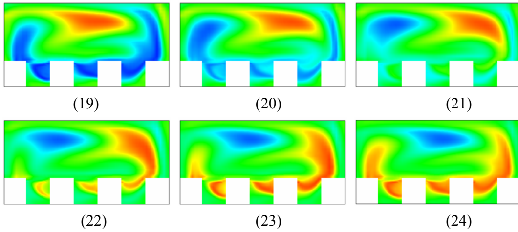
圖 4-37 SRM \alpha = 30^\circ ，下游 1~2cm 之間截面濃度分佈
