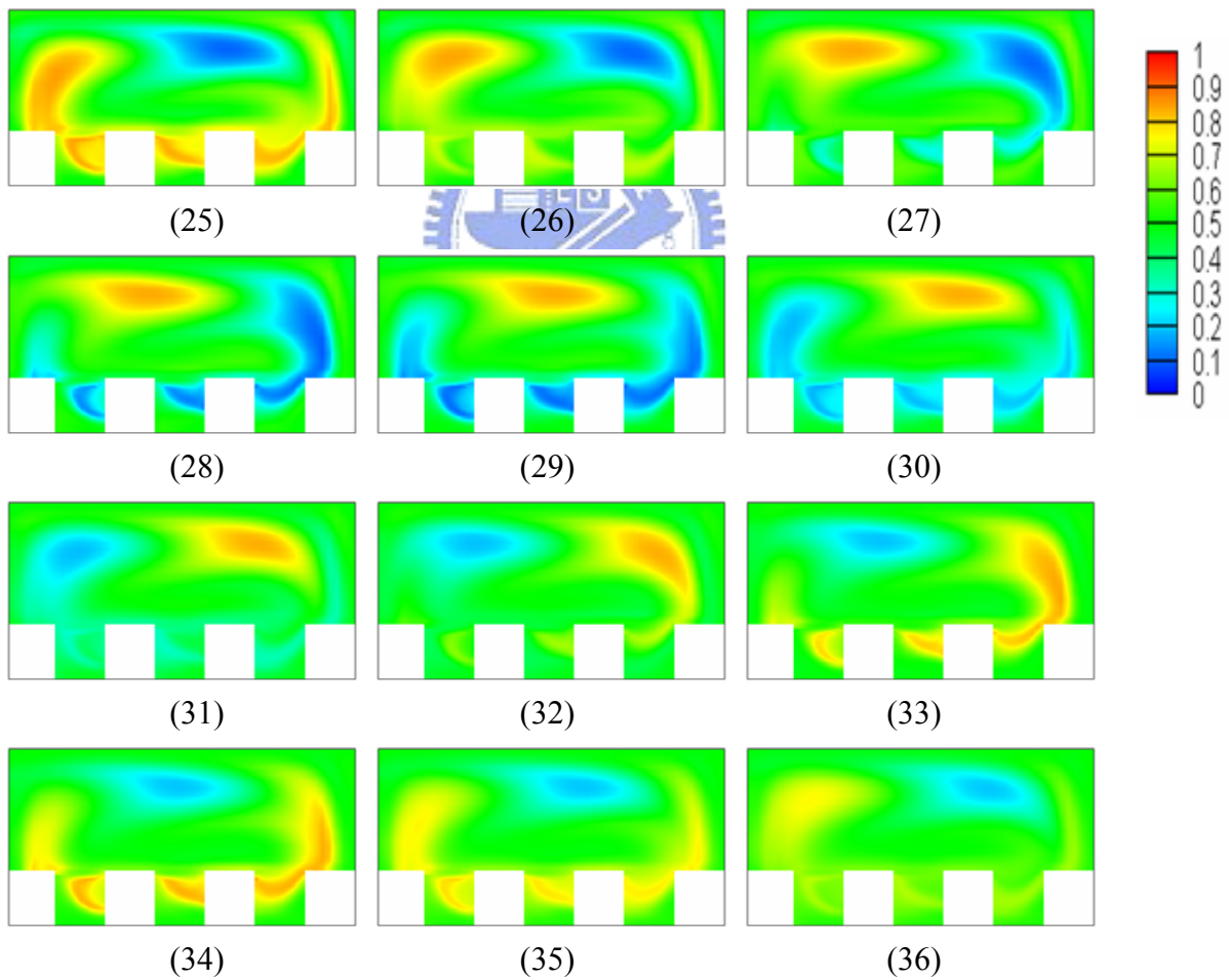
圖 4-38 SRM \alpha = 30^\circ ，下游 2~3cm 之間截面濃度分佈
