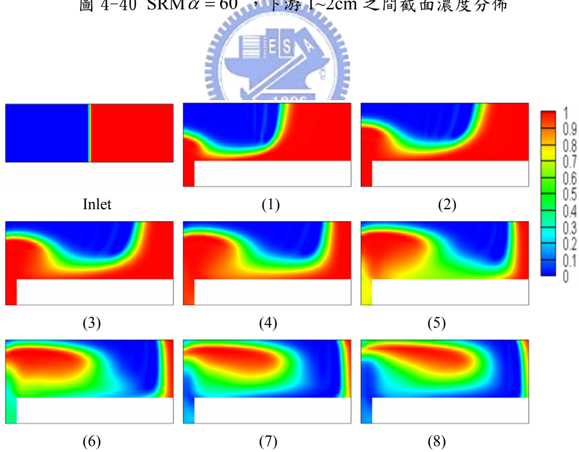
圖 4-40 SRM \alpha = 60^\circ ，下游 1~2cm 之間截面濃度分佈
