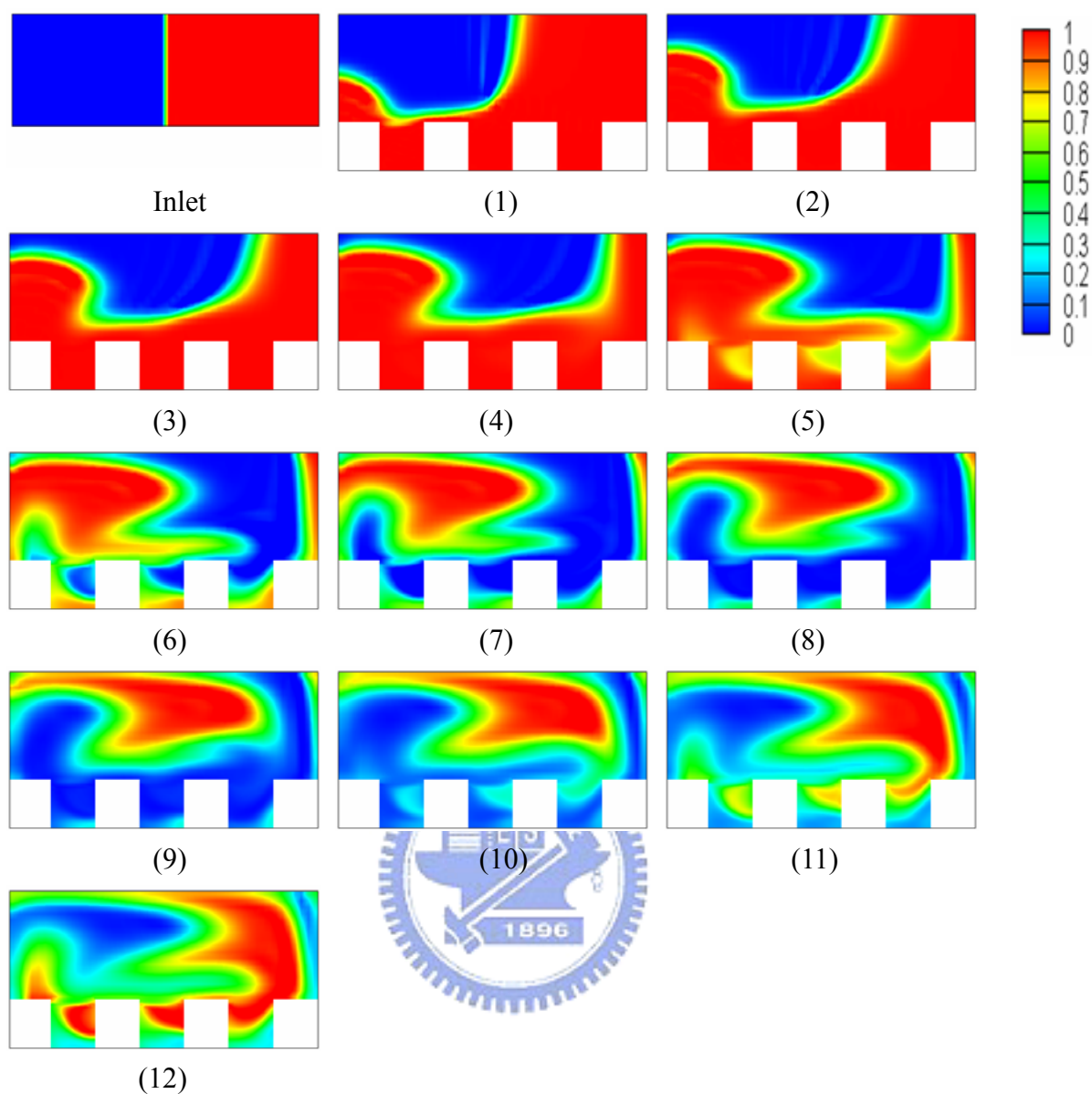
圖 4-36 SRM \alpha = 30^\circ 從入口到 1cm 之間截面濃度分佈
