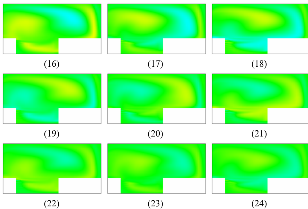
圖 4-40 SRM \alpha = 60^\circ ，下游 1~2cm 之間截面濃度分佈
