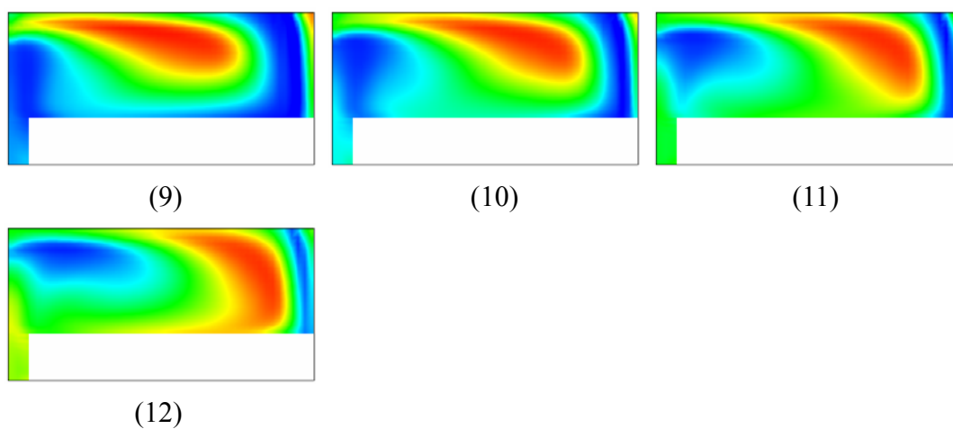
圖 4-41 SRM \alpha = 75^\circ ，從入口到 1cm 之間截面濃度分佈
