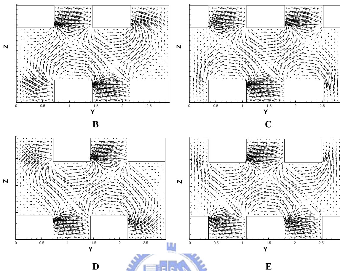
圖 4-47 Double SRM 於位置 B~E 的截面速度場
