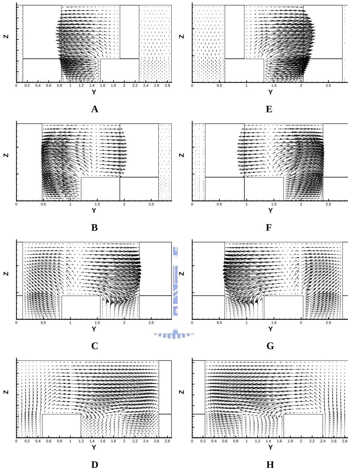
圖 4-58 OBSHM 於位置 A~H 截面速度場
