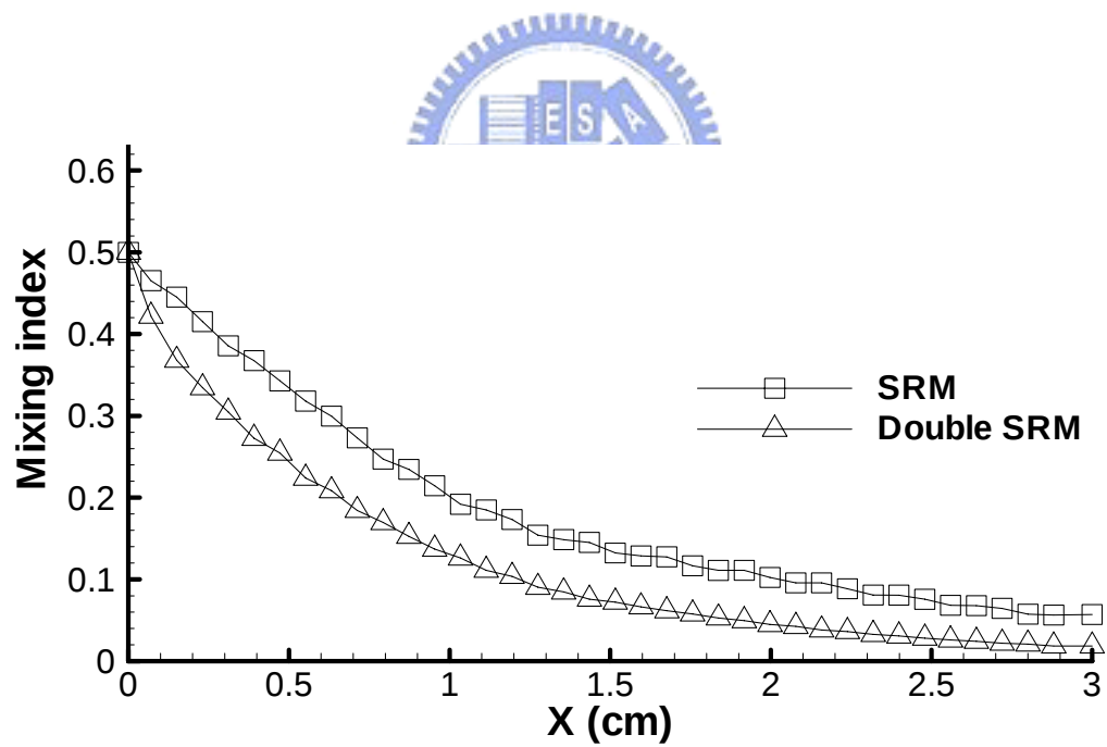
圖 4-50 單邊及上下壁面具斜凹槽混合指數比較
