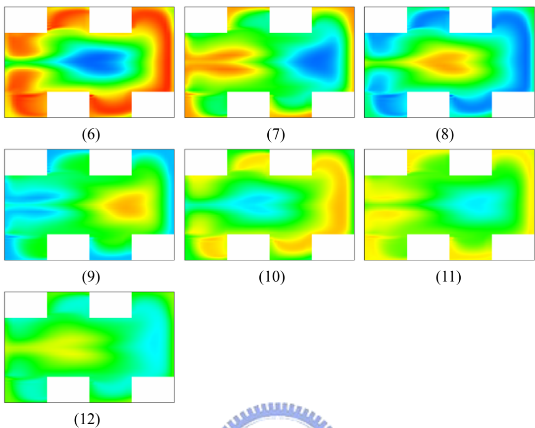
圖 4-48 Double SRM 入口到 1cm 之間截面濃度分佈
