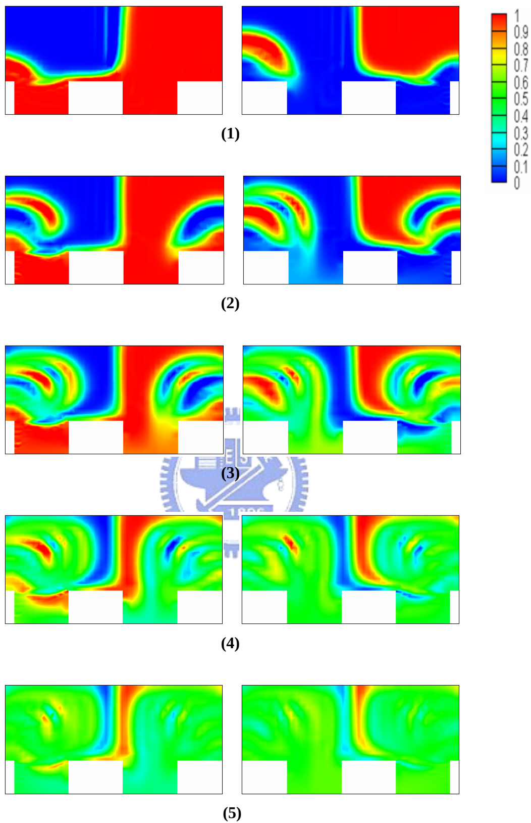
圖 4-54 SHM 從入口到 1cm 之間 C 及 G 截面濃度分佈
