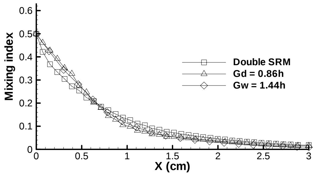
圖 4-51 Double SRM 和凹槽加深及加寬混合指數比較
