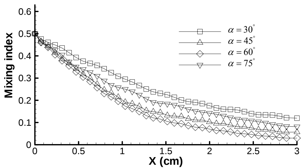
圖 4-44 SRM 於 Pe = 2 \times 10^5 時凹槽傾角 \alpha 對混合指數的
