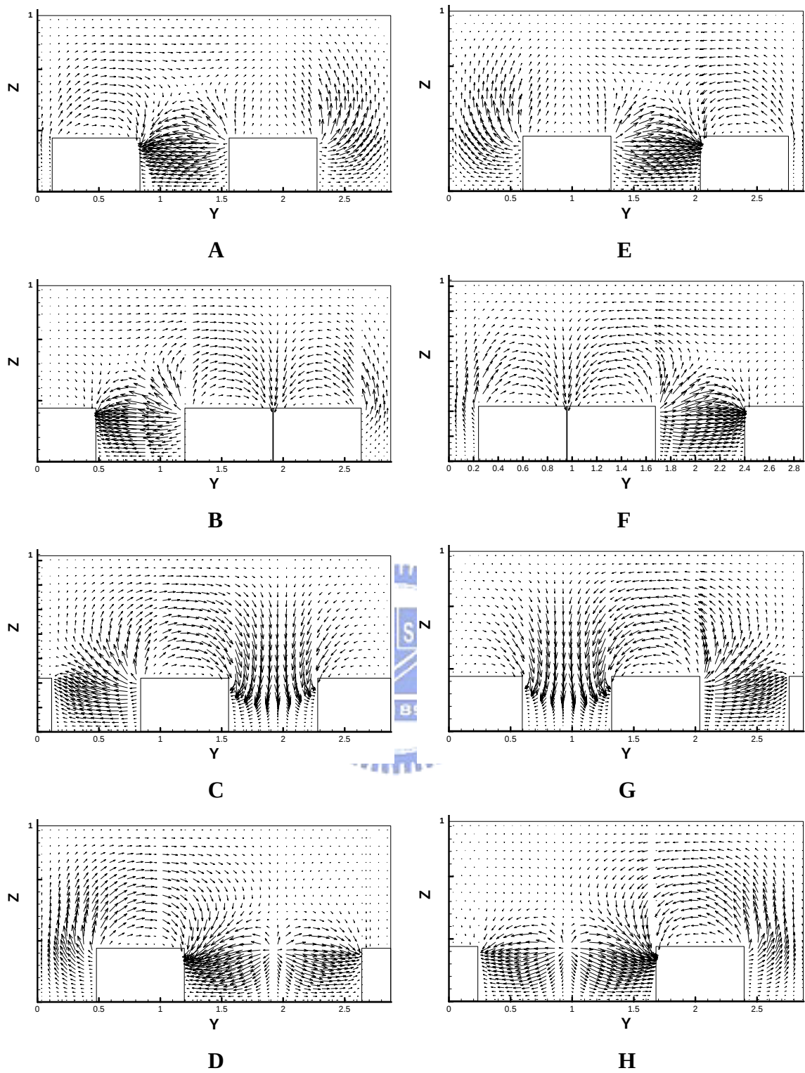
圖 4-53 SHM 於位置 A~H 截面速度場
