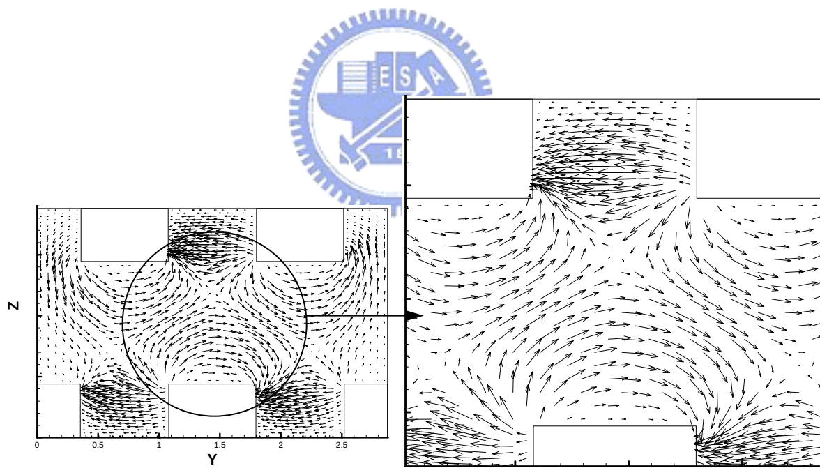
圖 4-46 Double SRM 於位置 A 的截面流場型態
