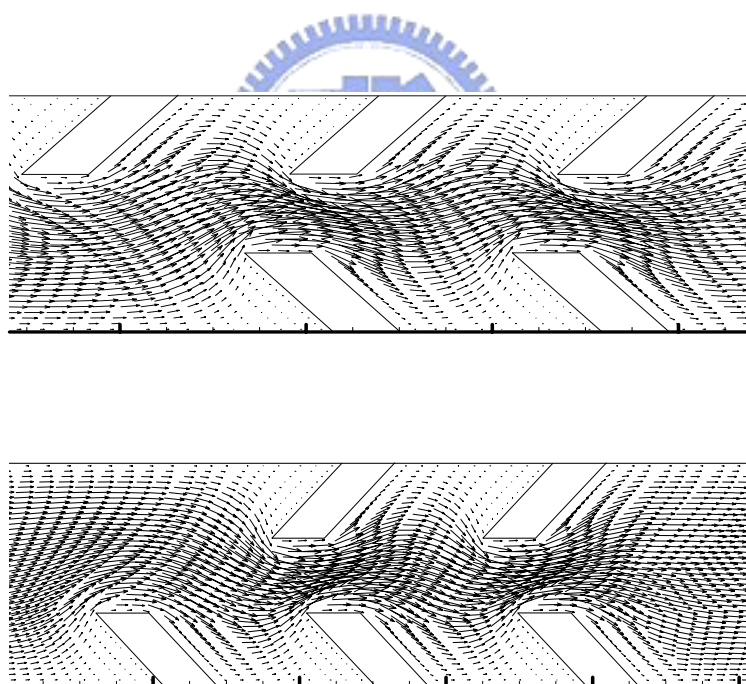
圖4-57 OBSHM 主流道中心截面速度場
