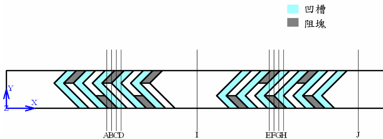
圖4-56 OBSHM 截面觀測位置示意圖
