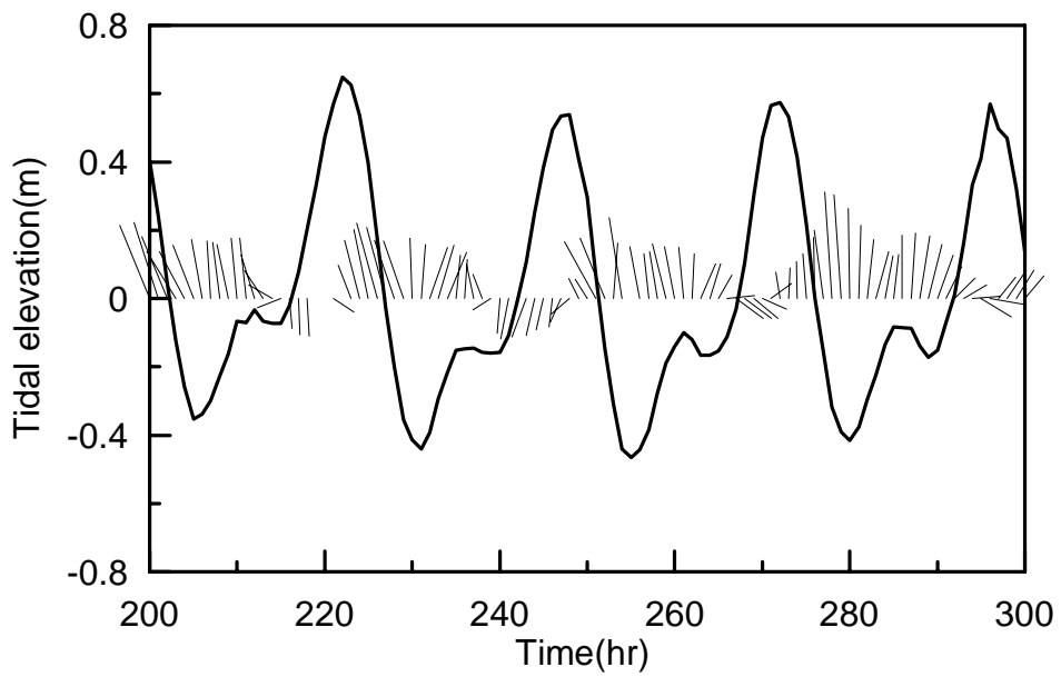
圖 4.1-12 高雄港 1 港口 2007/08 日潮不等大
