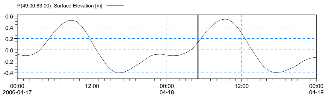
圖 4.4-4 高雄港附近海域潮流分布，參考潮位：高雄港，2006/04/18 05:00:00
