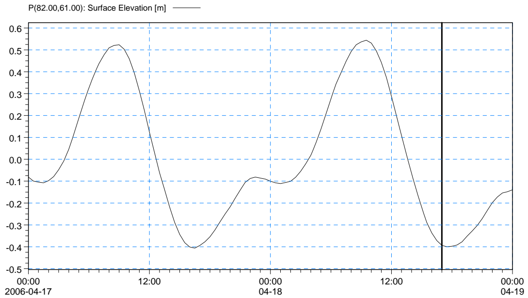
圖 4.3-14 高雄附近海域潮流分布，參考潮位：高雄港，2006/04/18 17:00:00
