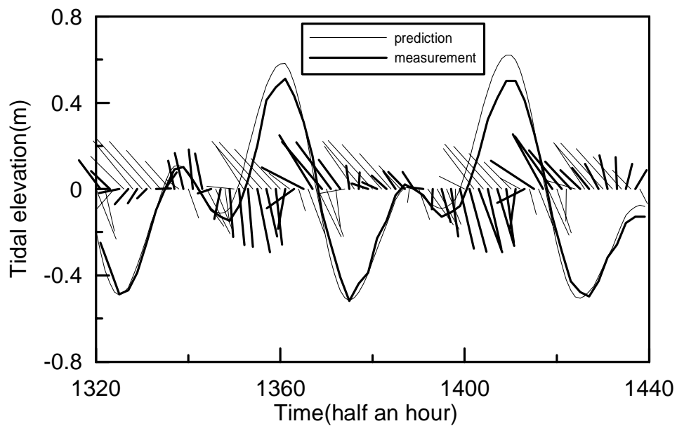
圖 4.4-8 高雄港附近海域潮位及潮流驗證(日潮不等大)
