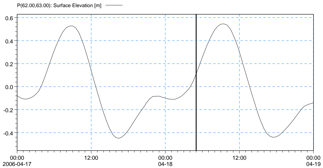
圖 4.2-4 臺灣附近海域潮流分布，參考潮位：高雄港，2006/04/18 05:00:00
