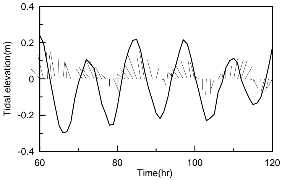
圖 4.1-11 高雄港 1 港口 2007/08 日潮不等小
