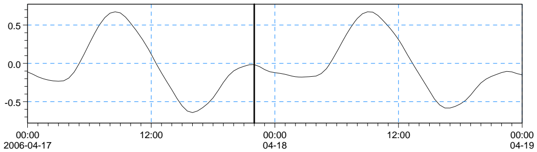
圖 4.3-2 臺灣南部海域潮流分布，參考潮位：高雄港，2006/04/17 22:00:00
