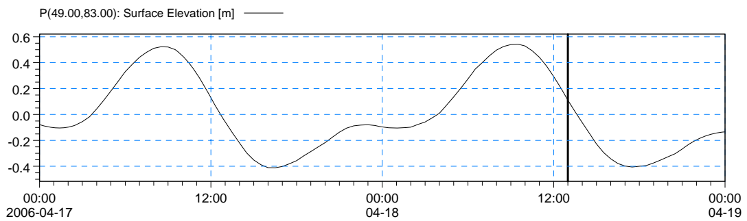
圖 4.4-6 高雄港附近海域潮流分布，參考潮位：高雄港，2006/04/18 13:00:00
