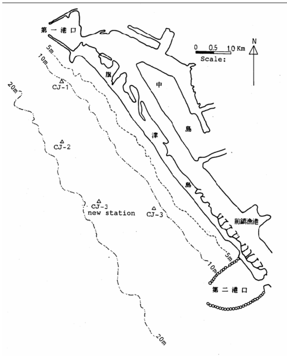
圖 2.2-1 旗津外海海流觀測作業位置圖
