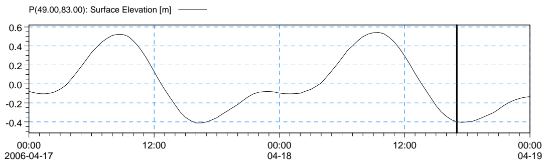
圖 4.4-7 高雄港附近海域潮流分布，參考潮位：高雄港，2006/04/18 17:00:00
