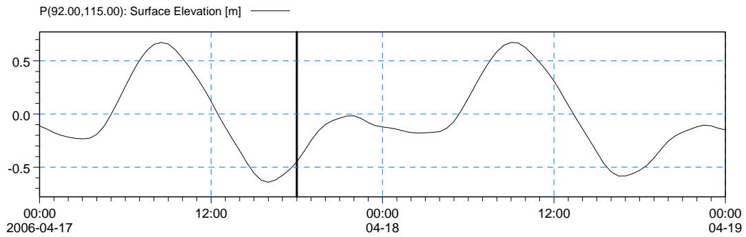
圖 4.3-1 臺灣南部海域潮流分布，參考潮位：高雄港，2006/04/17 18:00:00
