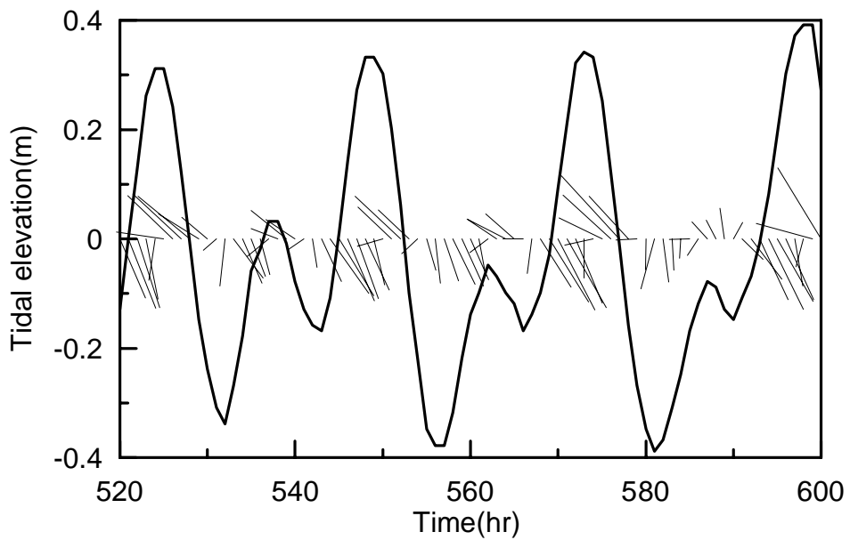
圖 4.1-4 高雄港 2 港口 2006/10 日潮不等大
