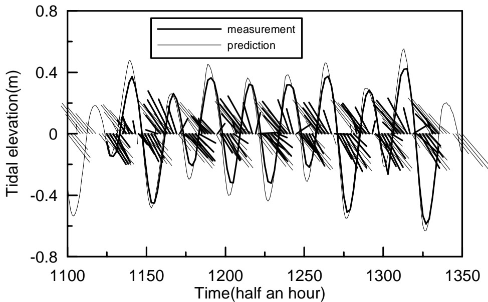
圖 4.2-8 大區域計算結果中安平港的驗證
